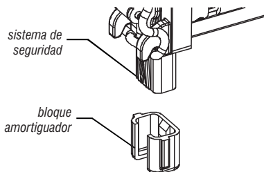
Fig. 10 – Bloque amortiguador;
