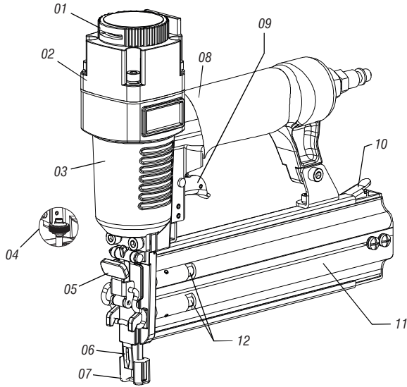
Fig.1 - Componentes del clavador
