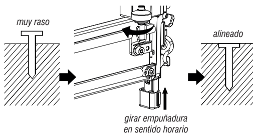
Fig. 7 – Clavos muy rasos
