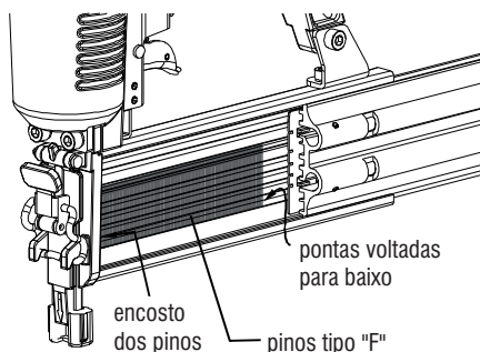
Fig. 4 – Posicionamento dos pinos
