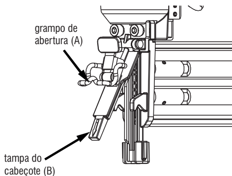
Fig. 11 – Abertura do cabeçote
