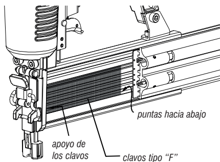
Fig. 4 – Posicionamiento de los clavos
