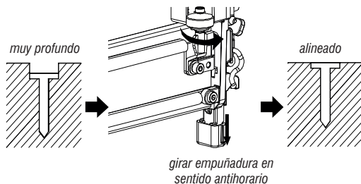
Fig. 6 – Clavos muy profundos
